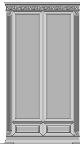
ШГ-2 ШКАФ ГЛУХОЙ РАЗМЕРЫ: выс./шир./гл. 2082x1104x477 мм
