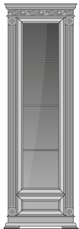
ШВ-1 ШКАФ ВИТРИНА РАЗМЕРЫ: выс./шир./гл. 2082x667x477 мм
