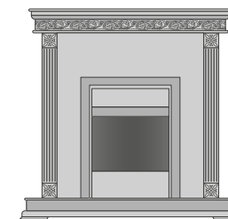
ШКм ПОРТАЛ ДЛЯ КАМИНА РАЗМЕРЫ: выс./шир./гл. 1080x1025x477 мм
