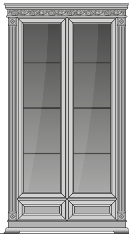
ШВ-2 ШКАФ ДВОЙНАЯ ВИТРИНА РАЗМЕРЫ: выс./шир./гл. 2082x1104x477 мм
