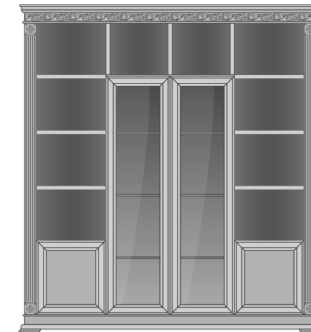
ШБ-3 ШКАФ РАЗМЕРЫ: выс./шир./гл. 2082x1903x477 мм
