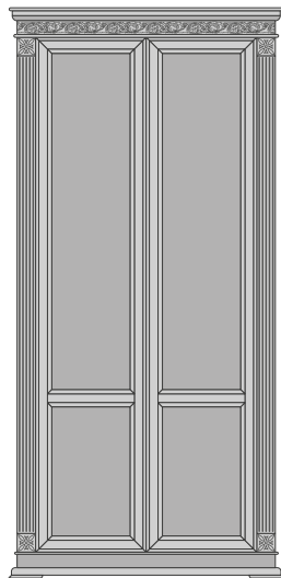
ШТГ-6 ШКАФ РАЗМЕРЫ: выс./шир./гл. 2282x1104x627 мм
