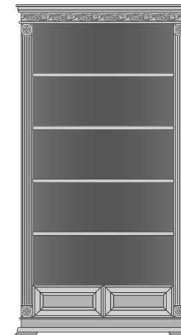
ШБ-2 ШКАФ РАЗМЕРЫ: выс./шир./гл. 2082x1105x477 мм
